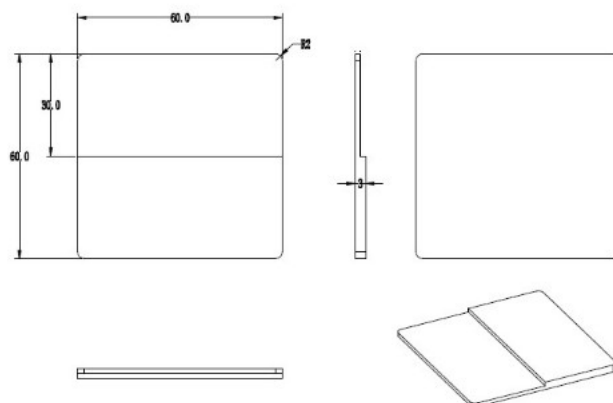
Double Door Striker
